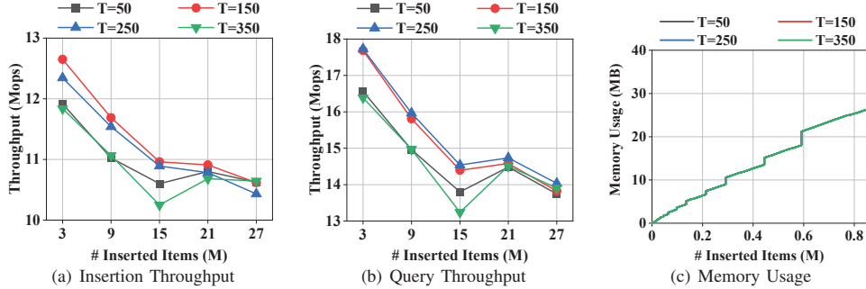
Fig. 4: Tuning experiments for parameter T .
