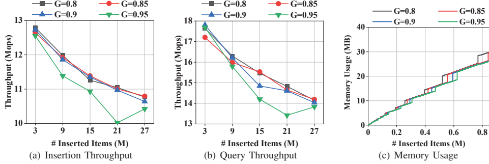
Fig. 3: Tuning experiments for parameter G .
