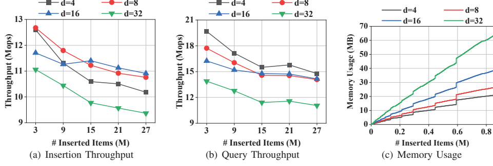
Fig. 2: Tuning experiments for parameter d .
