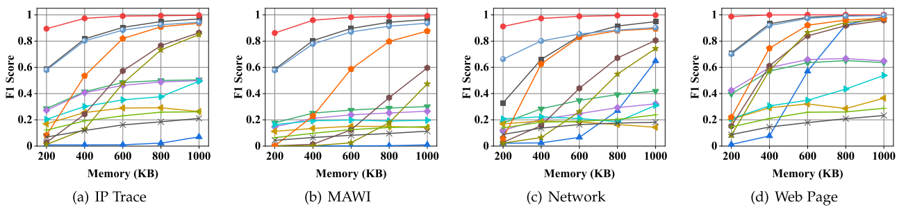
Fig. 11. F1 Score of heavy hitters.
